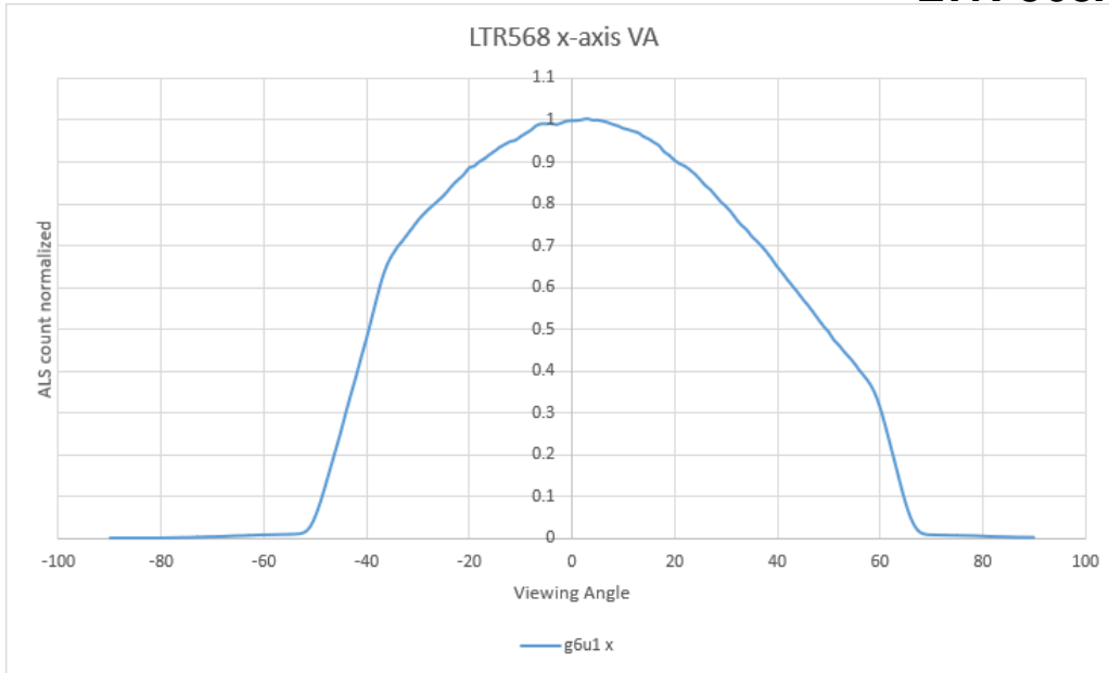
Figure 4.3: ALS viewing angle performance (X-axis)
