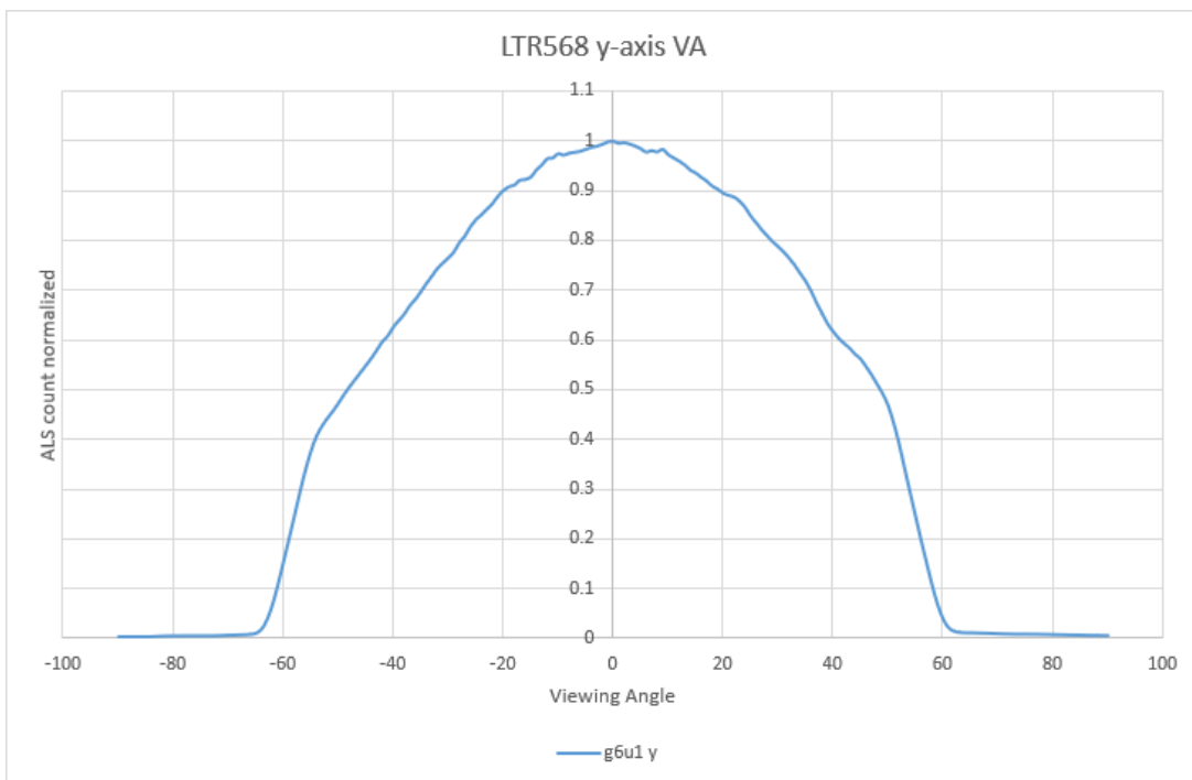
Figure 4.5 ALS viewing angle performance (Y-axis)
